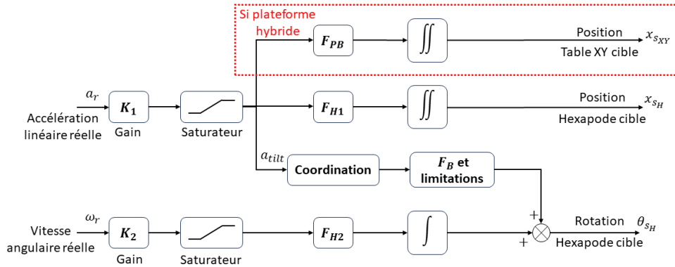
Figure 7.29 – MCA classique pour un mouvement longitudinal appliqué à une plateforme de Gough-Stewart (normal ou hybride).
