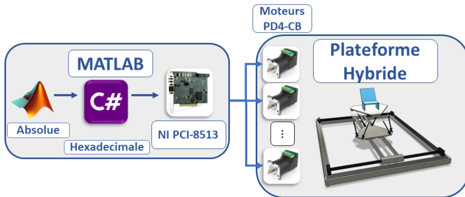
Figure 8.3 – Architecture système de la plateforme hybride.
