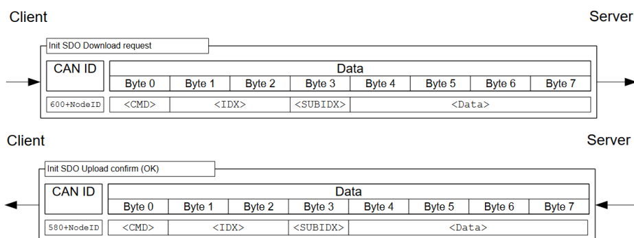
Figure 8.4 – Communication via le service SDO (émission en haut et réception en bas).
