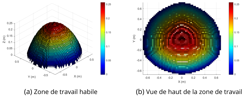
Figure 8.8 – Zone de travail habile de la plateforme parallèle de Gough-Stewart.
