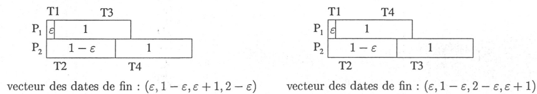
FIG. 4.4 – Exemple dans lequel c_{SPT}^*(\mathcal{I}) tend vers 2 quand \epsilon tend vers 0. Le nombre à l'intérieur de chaque tâche représente sa longueur, et l'inscription T_i à côté d'une tâche indique la tâche i .
