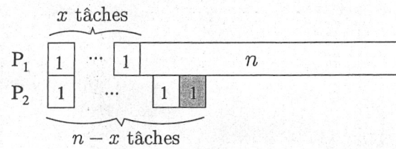
FIG. 5.7 – Ordonnancement (1 + \frac{x}{n}) -approché et équilibre de Nash (\frac{n-x}{x+1}) -approché.
