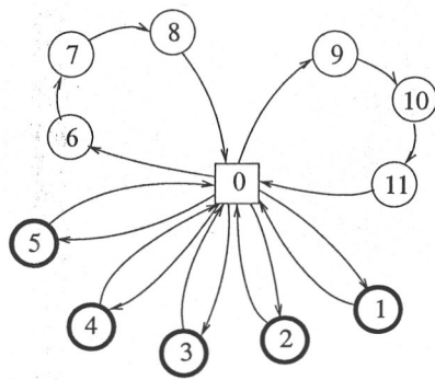
FIG. 3.6 – Les sommets mobiles sont les sommets 1 à 5. Le sommet mobile i a une demande égale à x_i . La meilleure solution voisine a un coût de 13 si et seulement si il existe une partition de \{x_1, x_2, x_3, x_4, x_5\} .
