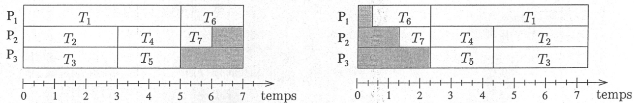
FIG. 6.3 – Gauche : Ordonnancement LPT. Droite : Ordonnancement LPT_{miroir} . T_i représente la tâche i .
