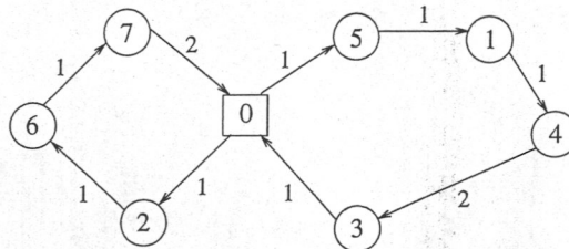
FIG. 3.4 – Une solution de coût 11 pour le PTV.
